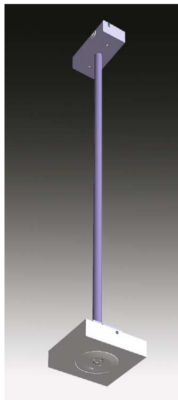
Optional Ceiling Bracket <1050mm long (for LEDLUX-SPOT3-A-P or B-P) Príplatková závesná konzola dĺžka <1050mm (pre LEDLUX-SPOT3-A-P alebo -B-P) Order Code: 182-B-201-01-00-01 (white RAL9003) Order Code: 182-B-201-01-00-02 (grey RAL9006)
